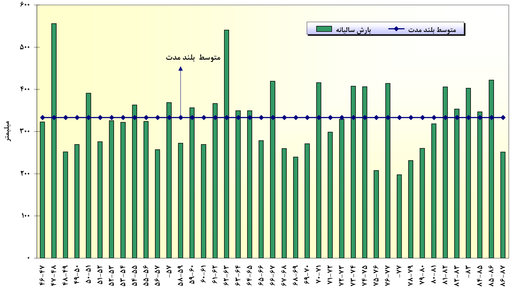
میزان بارش سالیانه استان تهران در دوره آماری ۴۱ ساله ( ۱۳۴۶-۸۷ )
